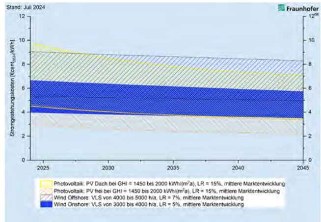
Abbildung 26: Entwicklung der Stromgestehungskosten für WEA und PV-Anlagen an Standorten mit hoher Windgeschwindigkeit (m/s) und Solarstrahlung kWh/(m 2 a).
